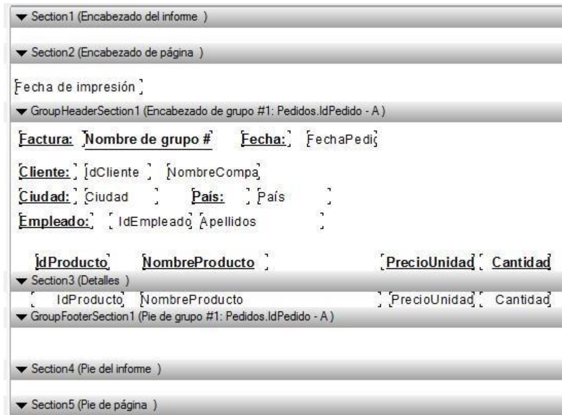
Diseñador de informe con tablas vinculadas mostrando campos relacionados.
