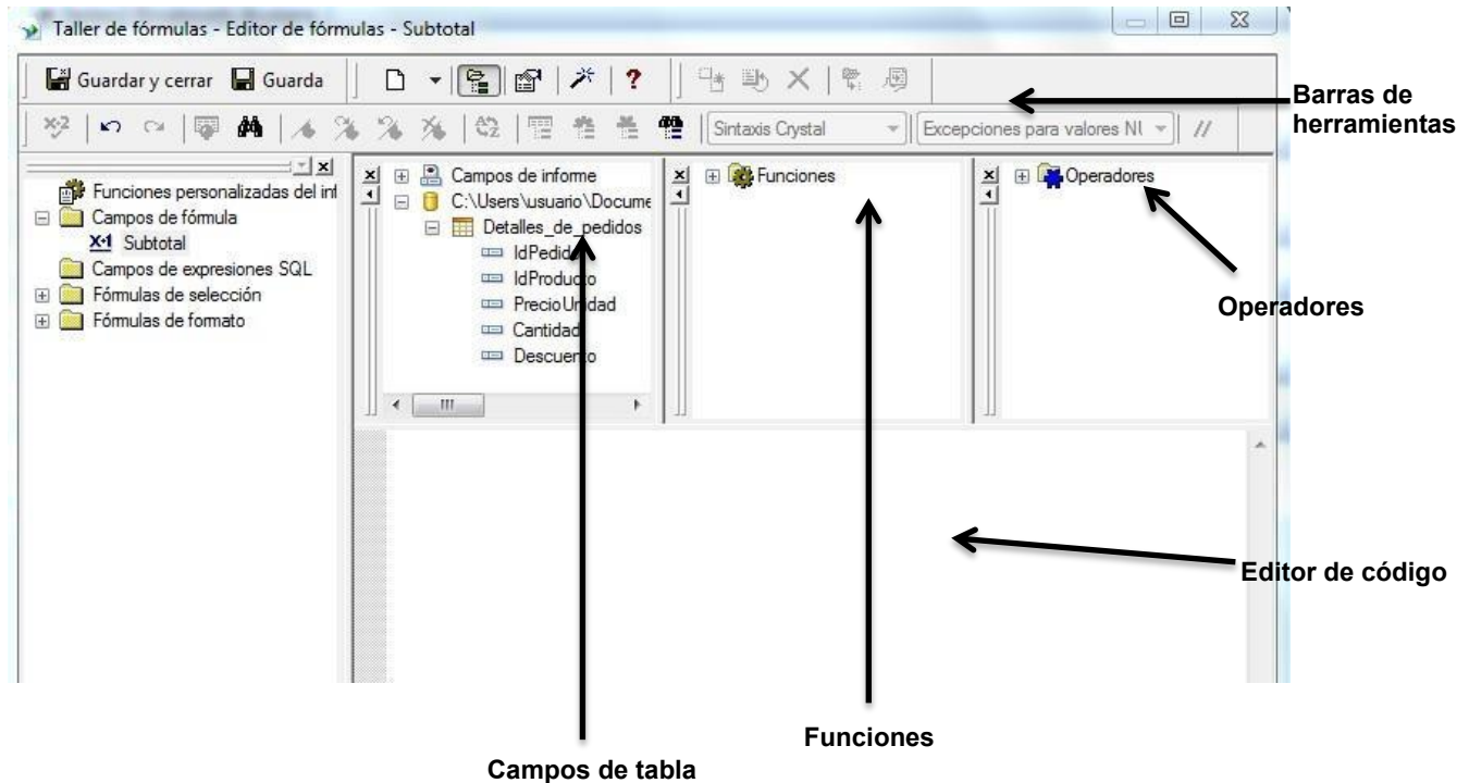
Ventana del editor de fórmulas.
